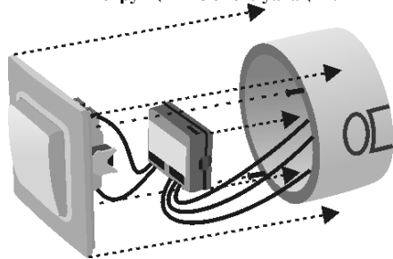
Рис. 1. Схема монтажа.
