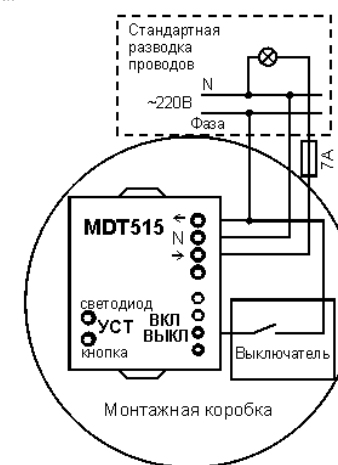
Рис. 3. Схема подключения модуля с нулем сети.
