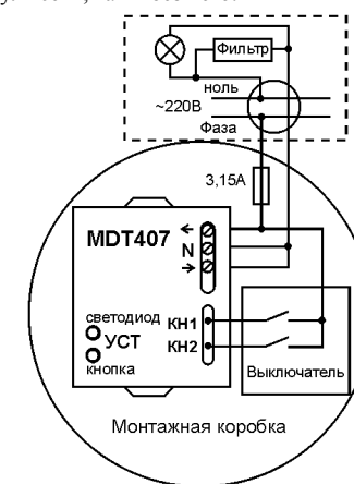
Рис. 2. Схема подключения модуля без нуля сети.
