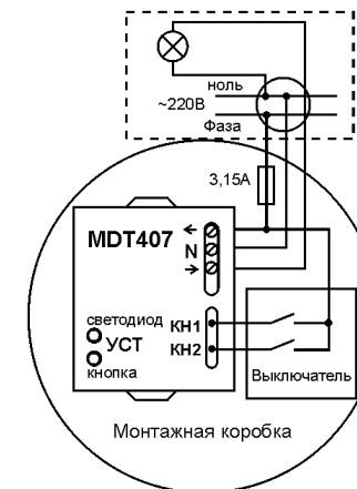
Рис. 3. Схема подключения модуля с нулем сети.
